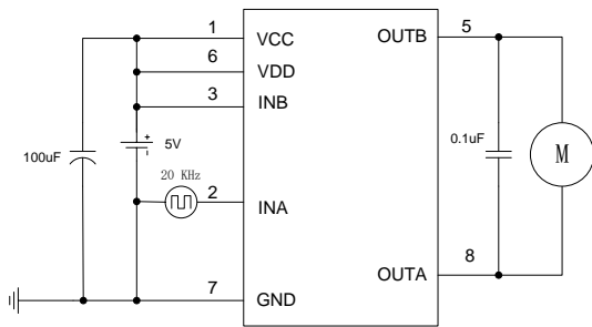
Time parameter test schematic
