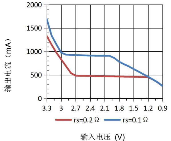
输出电流 vs. 输入电压
