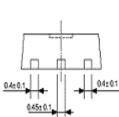
SOT89-3
