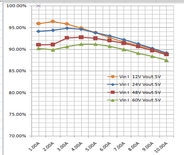
Fig. 4 效率曲线
